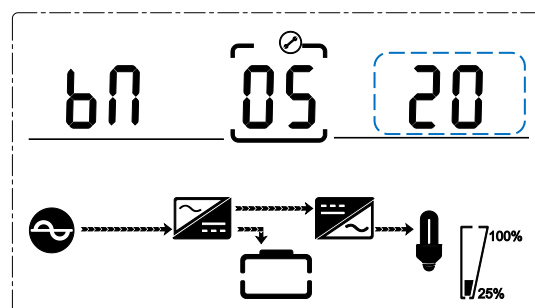
Fig. 4-17 Ajuste de la cantidad de baterías
