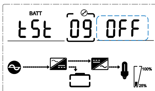
Fig. 4-21 Ajuste del autotest de la batería
