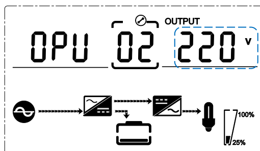
Fig. 4-14 Ajuste de la tensión de salida
