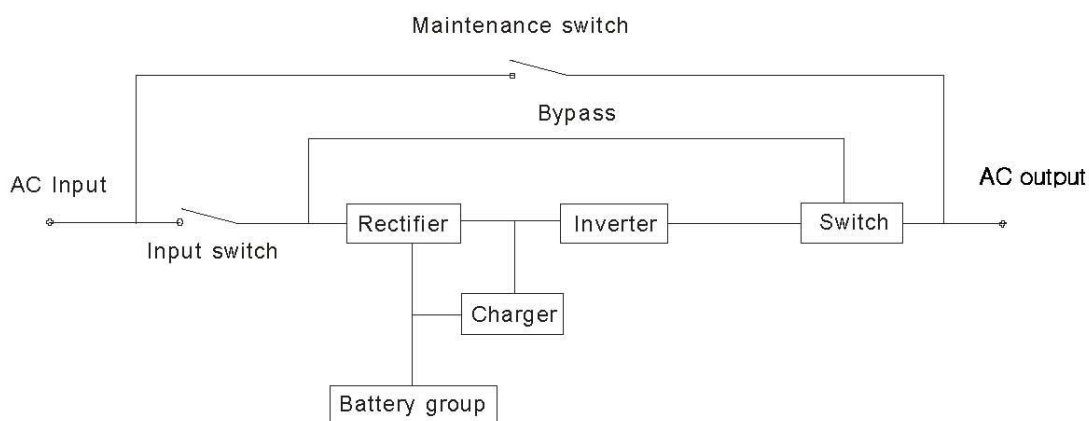
Fig. 2-1 Diagrama del ZGR EFFICIENT R 6 - 10 KVA
