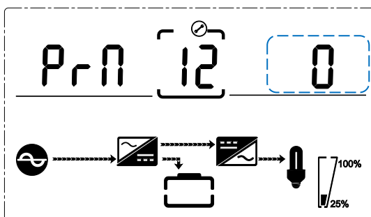
Fig. 4-27 Ajuste de la cantidad de redundancia paralela
