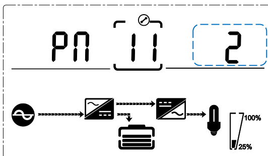
Fig. 4-26 Ajuste de la cantidad paralela
