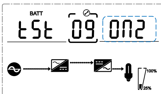
Fig. 4-23 Tiempos de autotest On2
