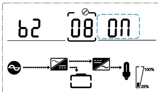
Fig. 4-20 Ajuste del zumbador de alarma
